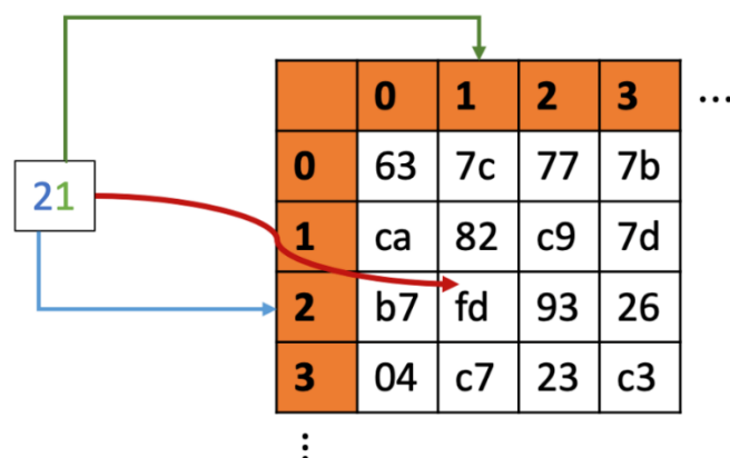
Fig. 2. Sustitución del valor 21 (hex) utilizando una caja de sustitución.
